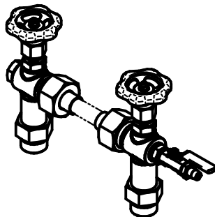
Fig.127 Ventilflüssigkeitsstand-Anzeiger Fig.127 Valve fluid-level indicator G1" -20°C / +200°C
