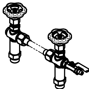
Fig.127 Ventilflüssigkeitsstand-Anzeiger Fig.127 Valve fluid-level indicator G3/4" -20°C / +200°C
