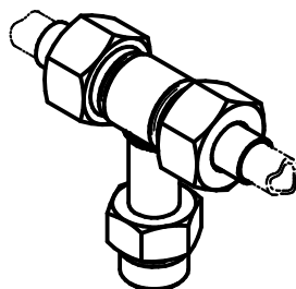
Fig.121 Zwischenhalter für Anzeiger Fig.121 Holder for fluid-level indicator G1" -20°C / +200°C
