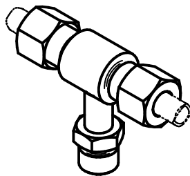
Fig.121 Zwischenhalter für Anzeiger Fig.121 Holder for fluid-level indicator G1/2" -20°C / +200°C
