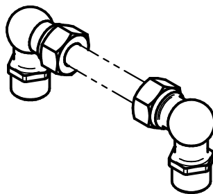
Fig.120/MS Flüssigkeitsstand-Anzeiger Fig.120/MS Fluid-level indicator G1/2" -20°C / +80°C
