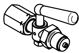
Fig.16 Manometer-Absperrhahn DIN 16262 A Fig.16 Manometer gauge cock DIN 16262 A G1/2" PN25 -10°C / +50°C
